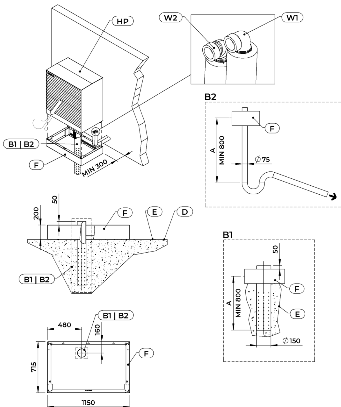
Abb. 26: ADAPT 2 auf einem Metallfundament TKT_ADAPT 2
