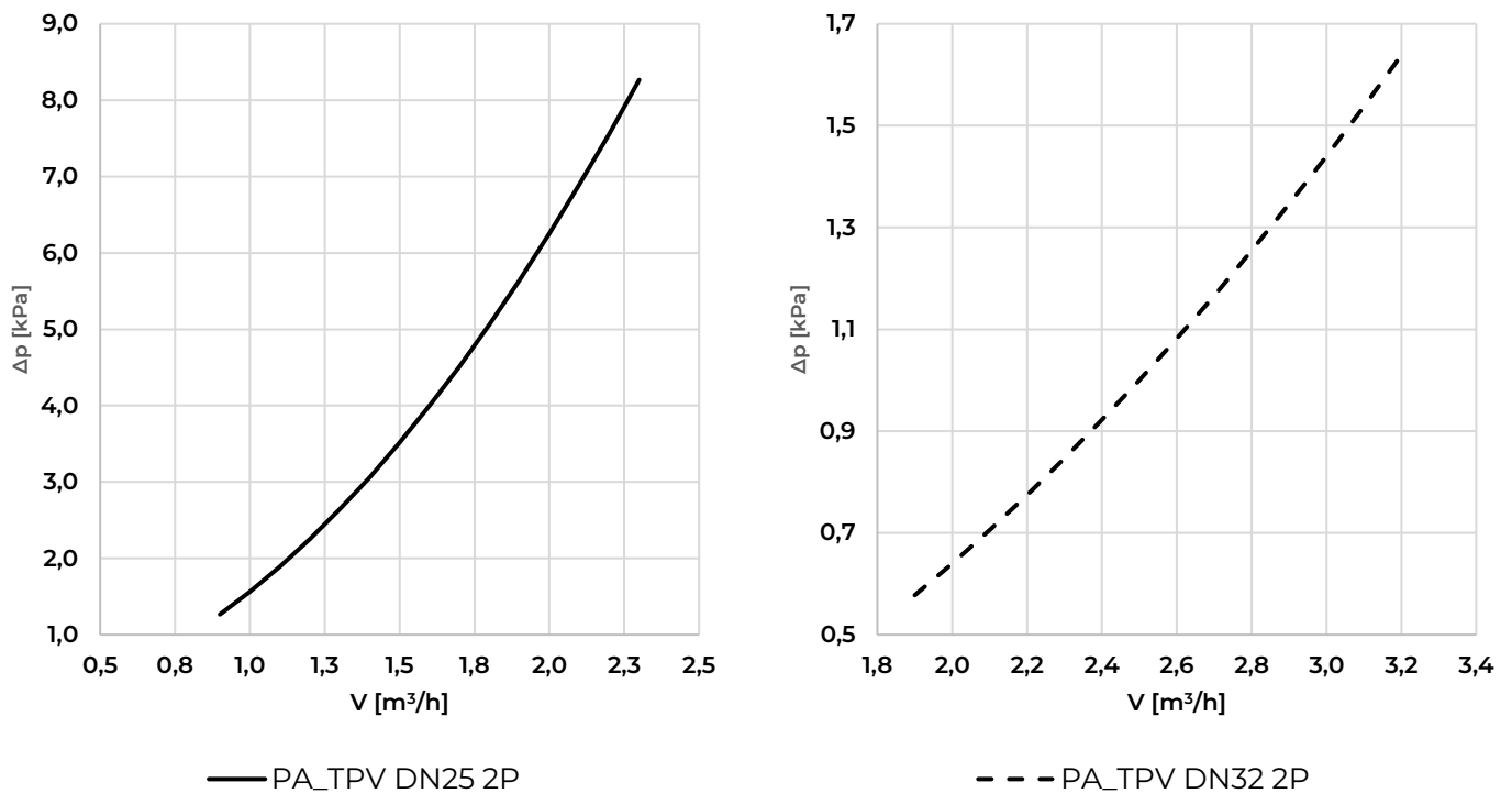
Abb. 22: Druckverlust für PA_TPV DN25 und PA_TPV DN32
