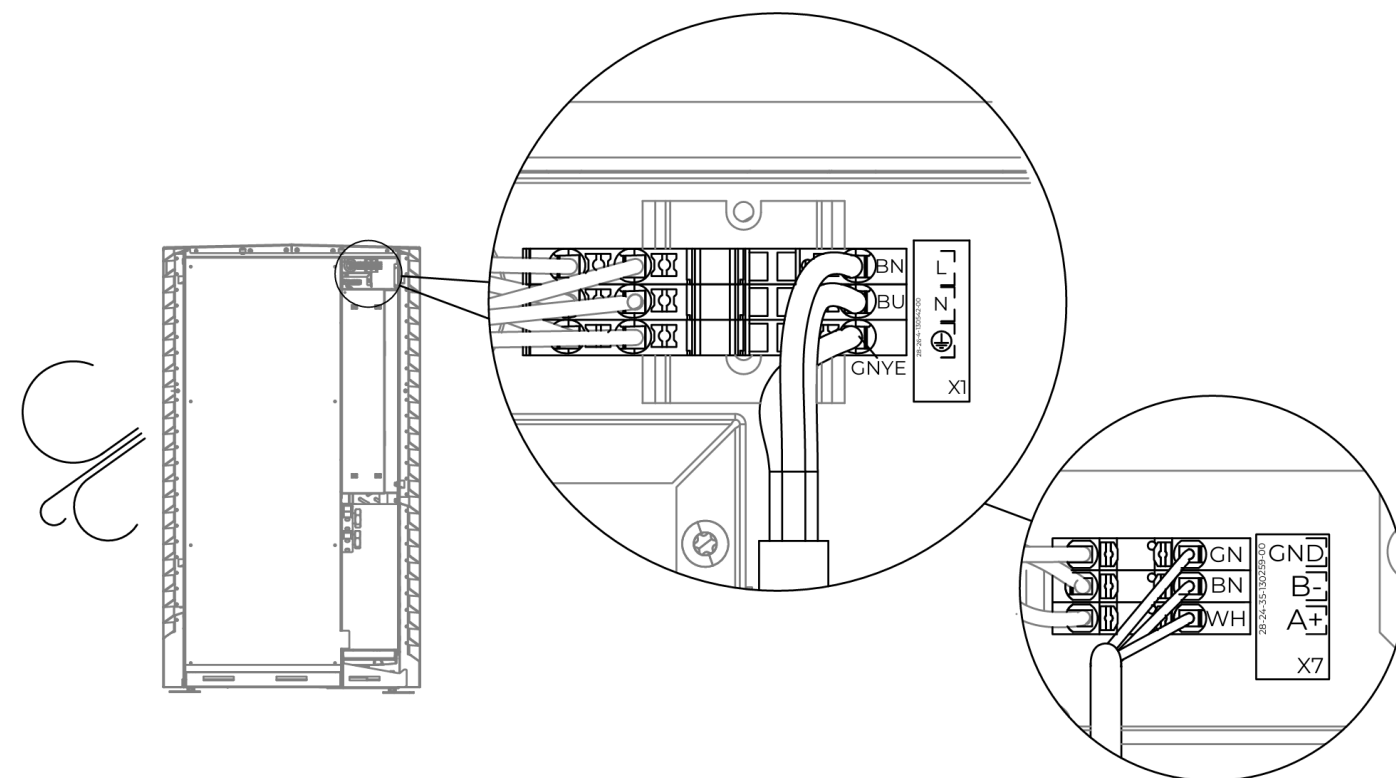
Abb. 52: Anschluss von Stromversorgung und Kommunikation für ADAPT 2 M 1F
