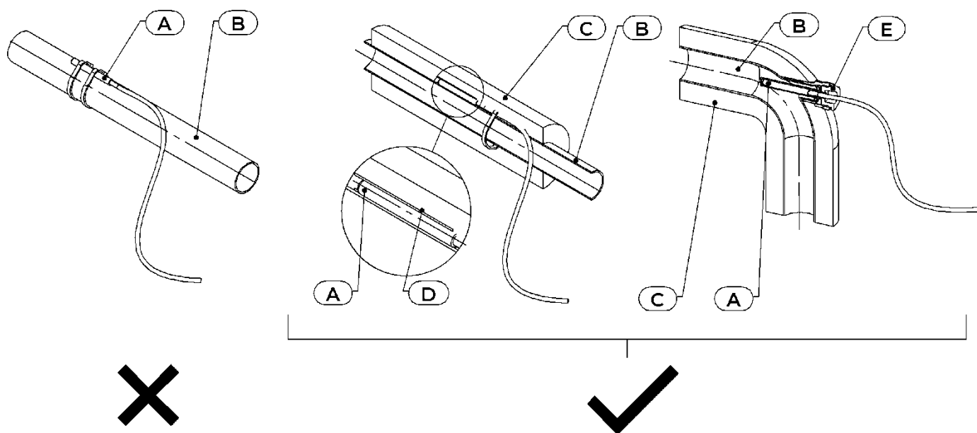
Abb. 27: Installation des Temperatursensors
