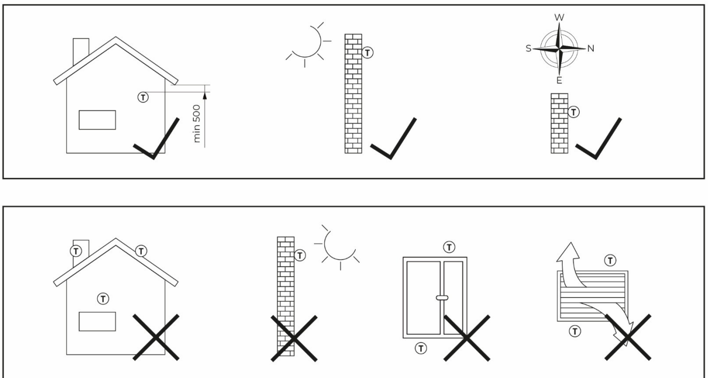
Abb. 36: Bestimmung der geeigneten Montageposition für den kabelgebundenen oder drahtlosen Außentemperaturfühler.
