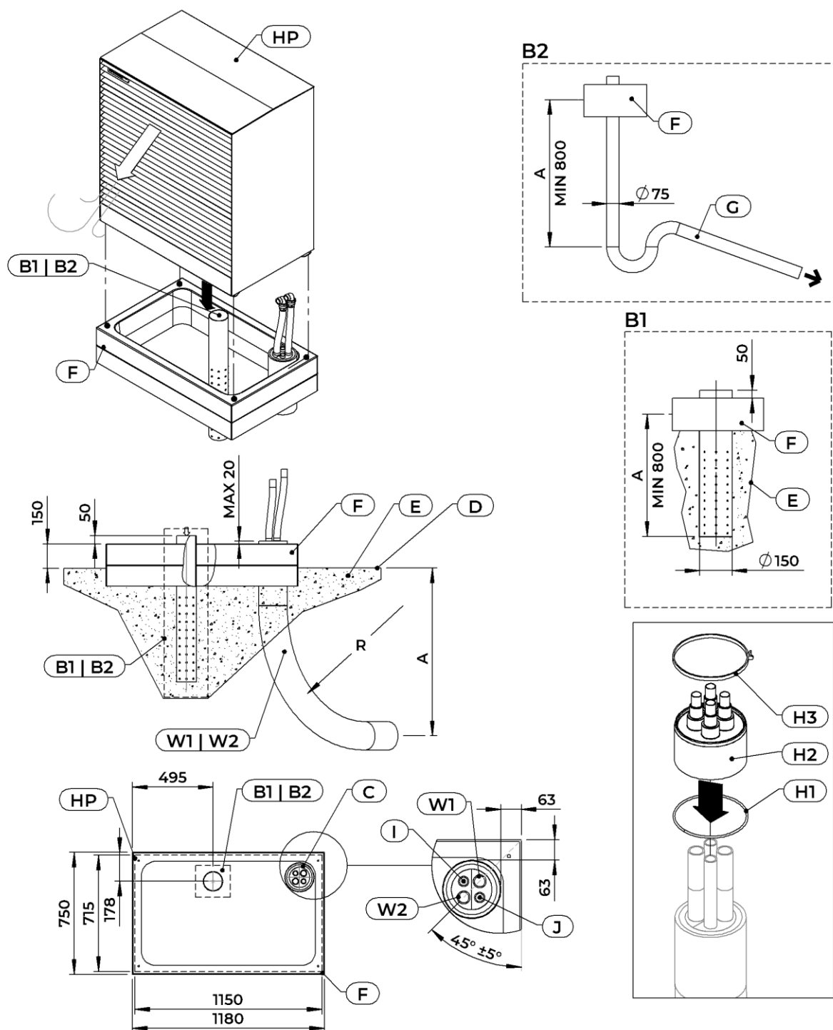
Abb. 25: Vorgefertigtes Betonfundament ZBT_ADAPT 2, Rohranschluss unterirdisch
