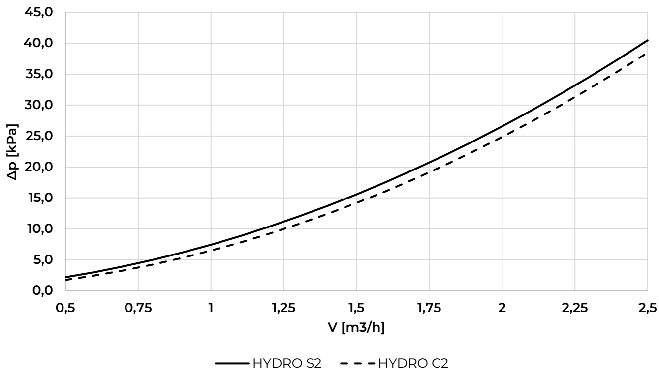
Abb. 20: Druckverlust für HYDRO S2 und HYDRO C2
