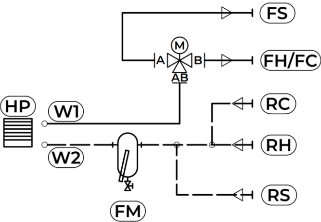
Abb. 32: Magnetischer Schlammabscheider im Rücklauf der Wärmepumpe installiert
