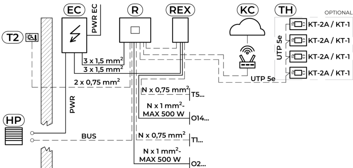
Abb. 35: Elektrisches Anschlussschema WR KSM 2 und WR KSM+
