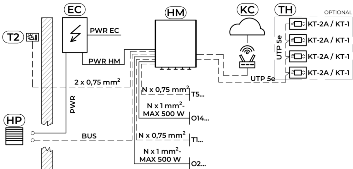
Abb. 34: Elektrisches Anschlussschema HYDRO S2
