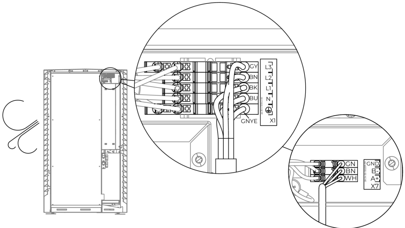
Abb. 53: Anschluss von Stromversorgung und Kommunikation für ADAPT 2 M/L 3F
