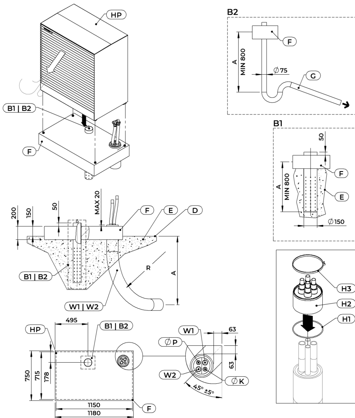
Abb. 23: Betonfundament ADAPT 2, Rohranschluss unterirdisch
