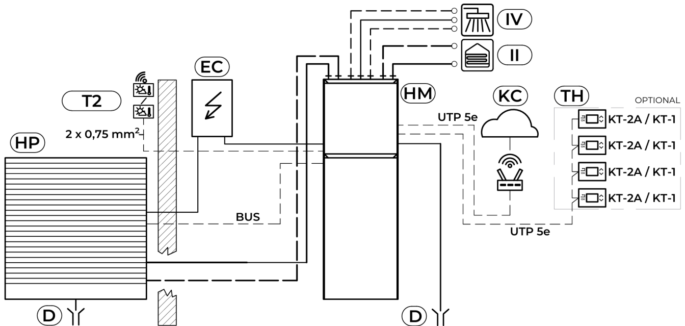
Abb. 2: Anschlusschema - ADAPT 2 + HYDRO C2
