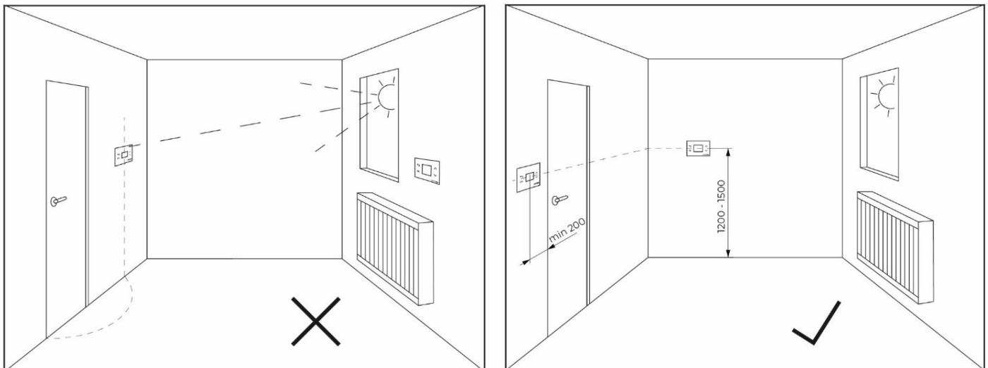
Abb. 38: Korrekte Installation des KT-2A Reglers und Thermostats
