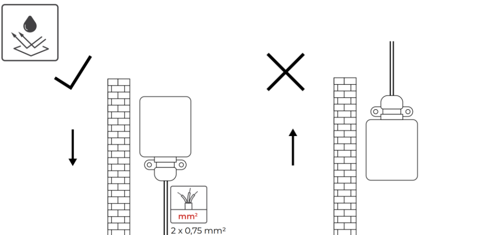
Abb. 37: Korrekte Ausrichtung bei der Montage des Außentemperaturfühlers
