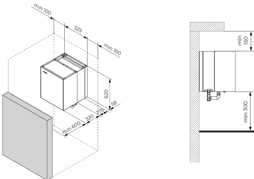
Abb. 16: Mindestfunktionsabstände für den Betrieb – HYDRO S2 + HYDRO P2 + HYDRO A2
