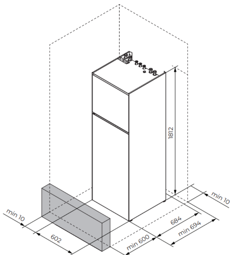
Abb. 12: Mindestfunktionsabstände für den Betrieb – HYDRO C2
