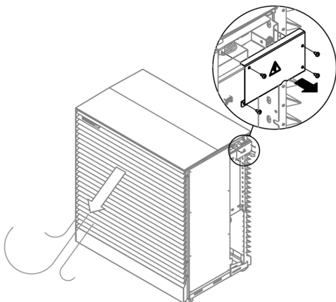
Abb. 50: Abnehmen der Schaltkastenabdeckung
