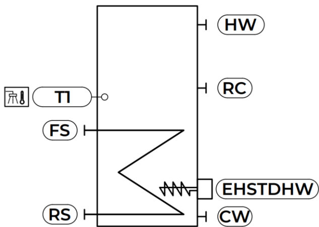
Abb. 29: Diagramm zur Installation von Sensoren im Warmwasserspeicher
