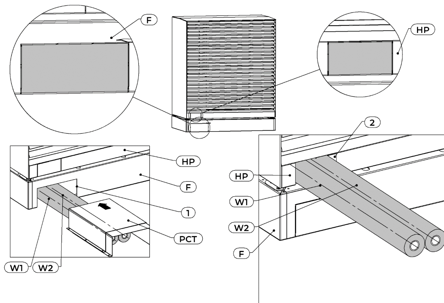
Abb. 49: Ausführung des Rohranschlusses durch den hinteren Teil der Wärmepumpe oder durch das Metallfundament TKT
