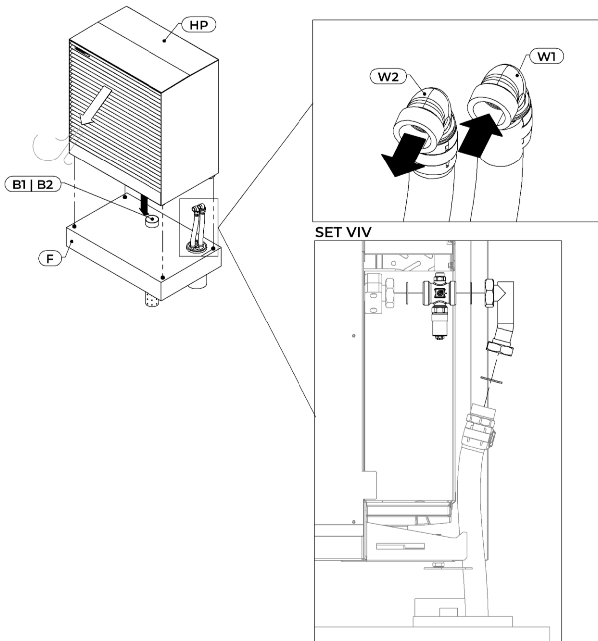
Abb. 47: Rohranschluss ADAPT 2
