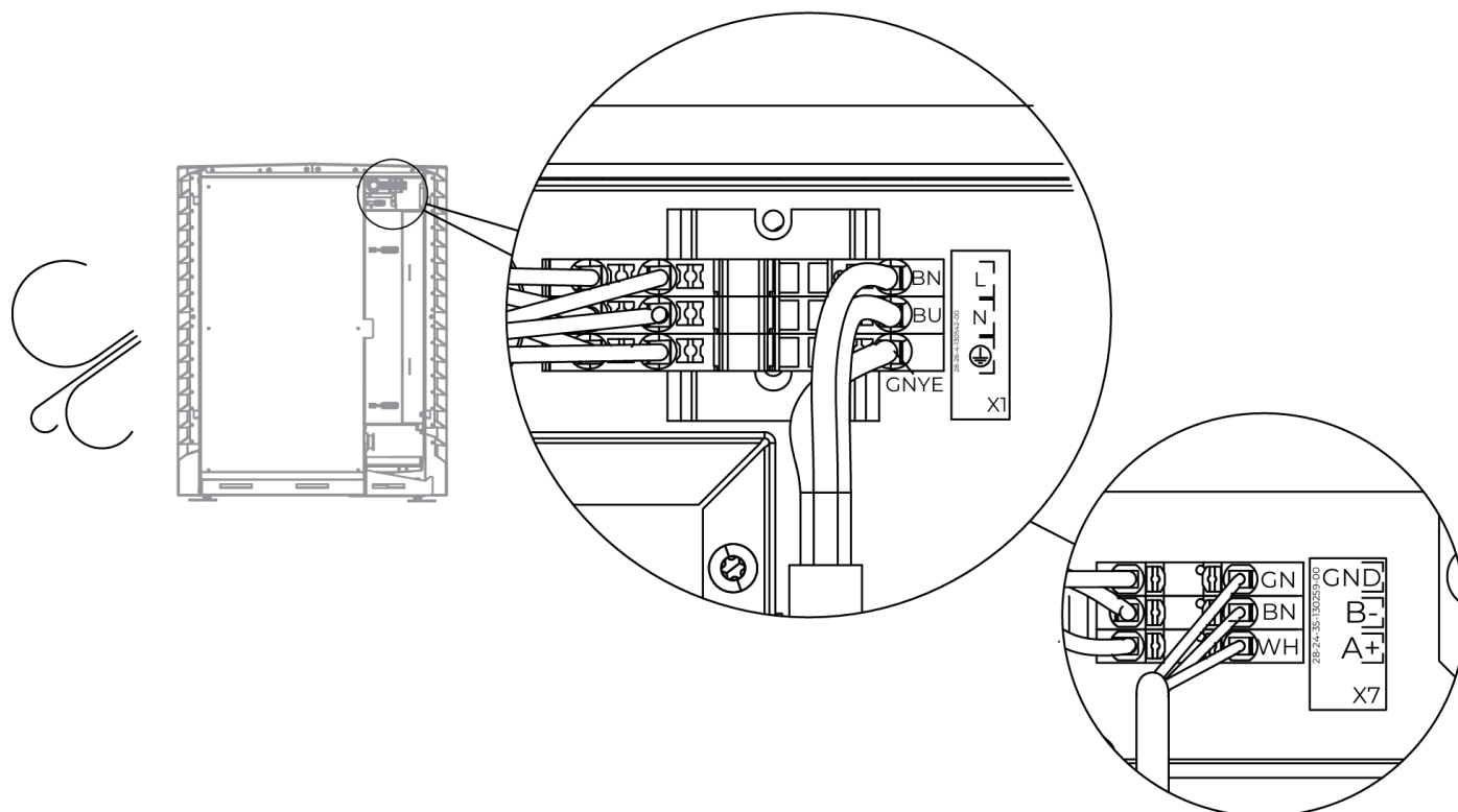
Abb. 51: Anschluss von Stromversorgung und Kommunikation für ADAPT 2 S 1F
