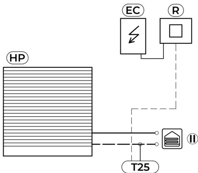
Abb. 28: Positionsschema des Drucksensors
