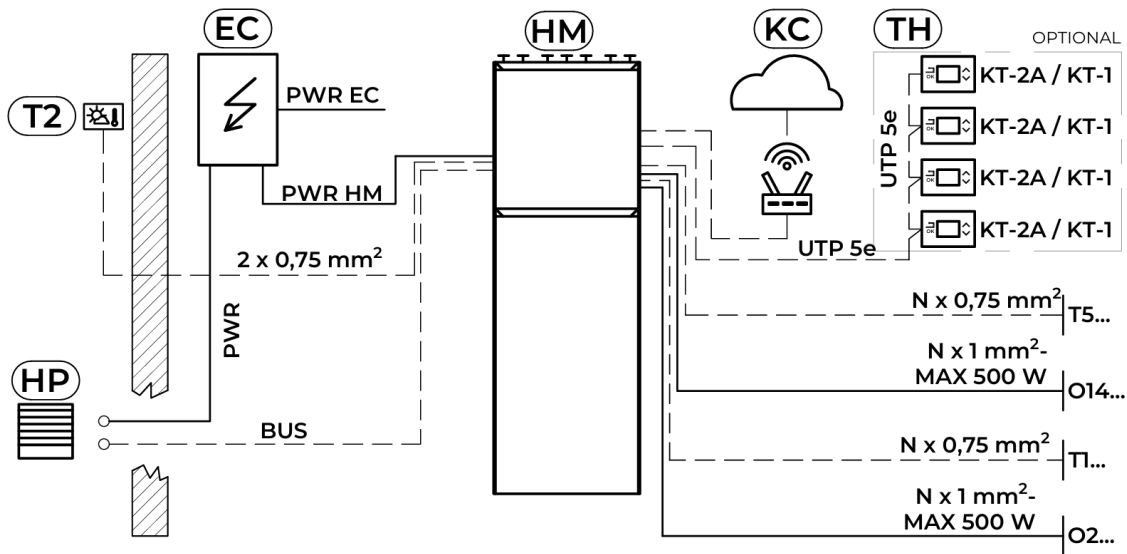
Abb. 33: Elektrisches Anschlussschema HYDRO C2
