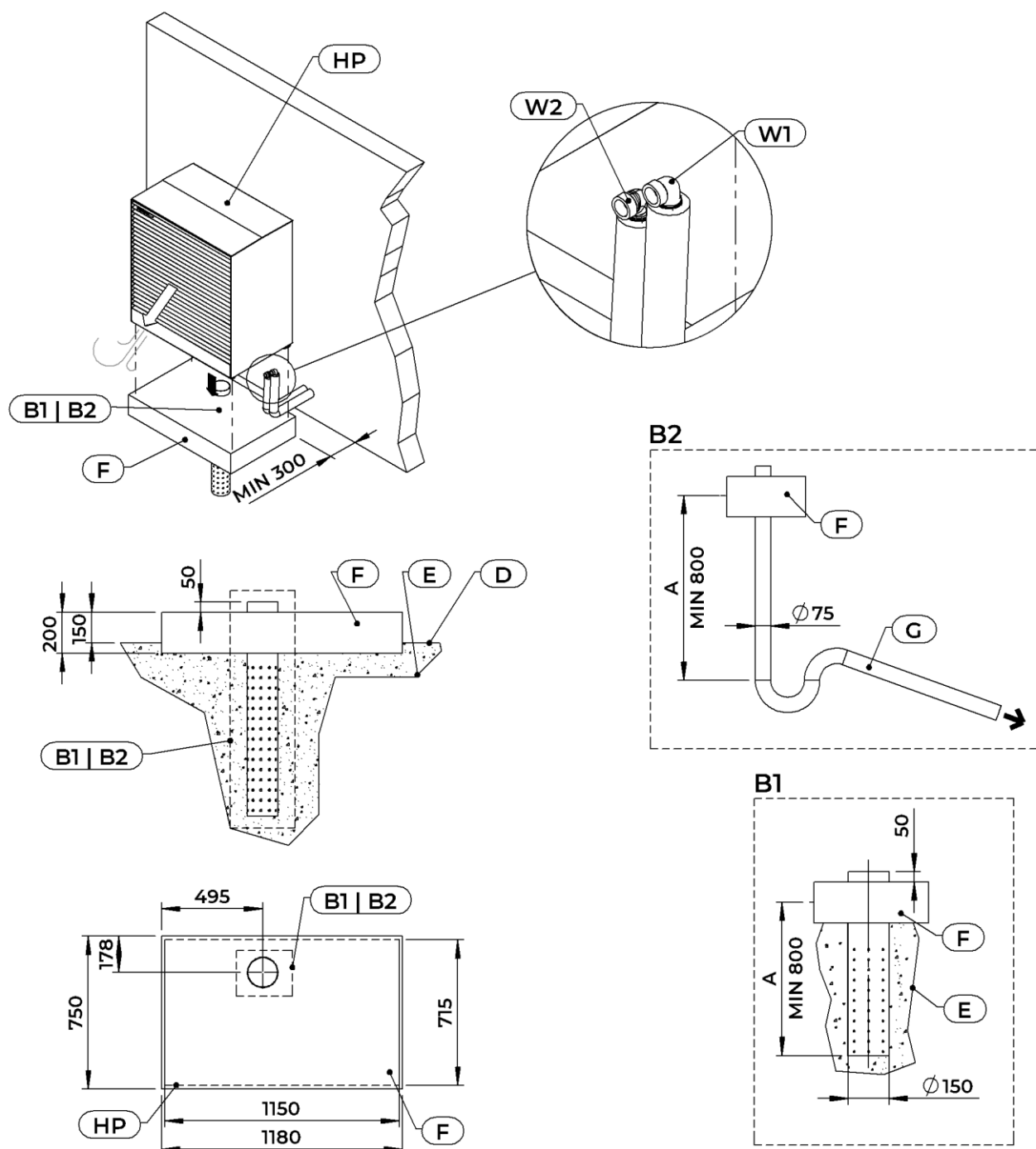
Abb. 24: Betonfundament ADAPT 2, Rohranschluss oberirdisch
