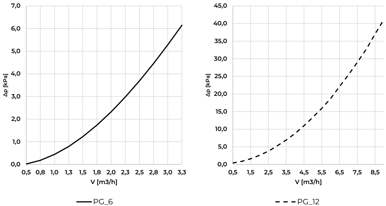
Abb. 21: Druckverlust für PG_6 und PG_12
