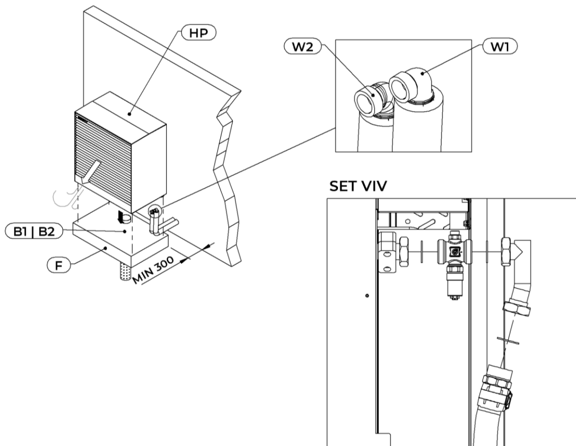
Abb. 48: Oberirdischer Rohranschluss
