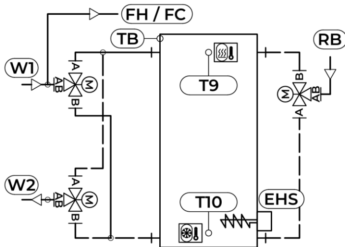
Abb. 31: Installationsdiagramm der Sensoren im Heiz- und Kühlepufferspeicher
